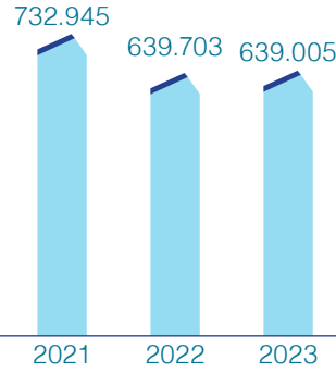
Toplam Su Çekimi (m³)
