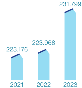
Atık Su Miktarı (m³)
