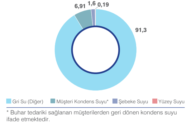
Kaynağına Göre Su Çekimi (%)
