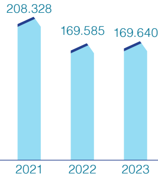
Sera Gazı Emisyonları (tCO 2 e) - Kapsam 1
