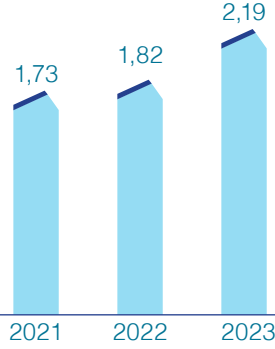
Doğal Gaz Çevrim Santrali Üretim Başına Su Tüketimi (m³/MWh)
