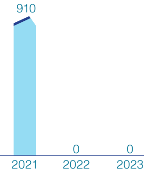
Sera Gazı Emisyonları (tCO 2 e) - Kapsam 2
