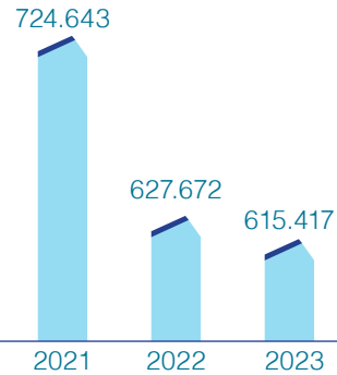
Geri Kazanılan/Tekrar Kullanılan Su Miktarı (m³)
